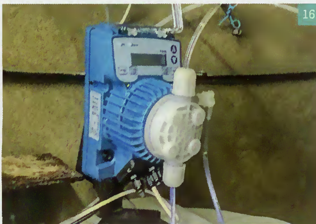
SISTEMA DE DESINFECÇÃO DE ÁGUA EM BARRAL, BALANÇA
