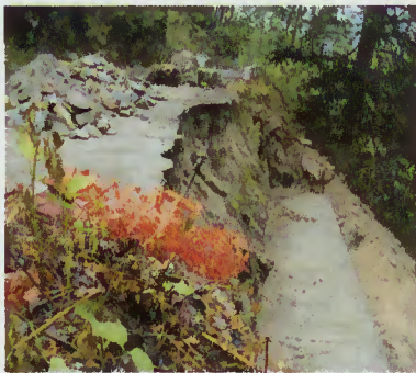
Construção do muro de suporte na estrada de Gerês- Portela do Homem
