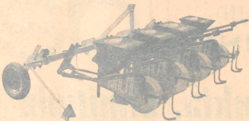
4 SEMEADORES «SIALAL» Ref.ª 604-TT, montados em barra Porta Alfaías, «SIALAL» Ref.ª 20-TT
