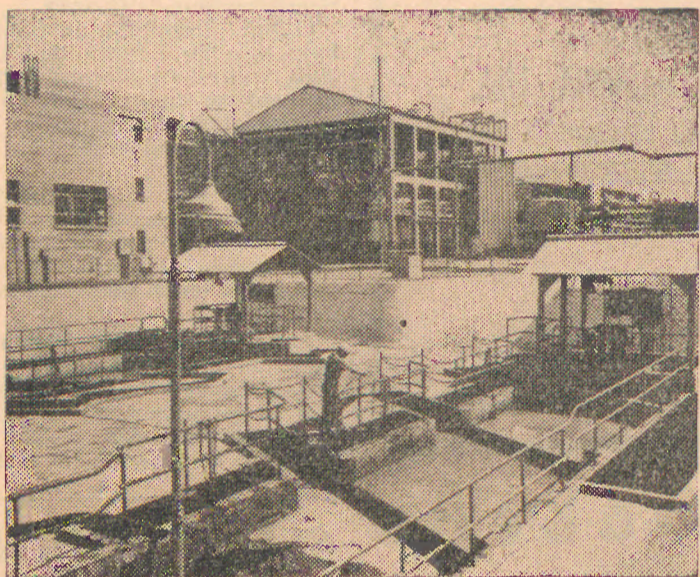
Aspecto da secção de polimerização da fábrica de Torrance, da Shell Chemical Corporativa
